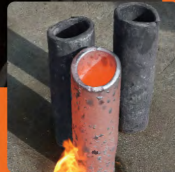
جنس: ۱-۷۲۲۵ قطر خارجی: ۸۳ میلی متر قطر داخلی: ۶۳ میلی متر ارتفاع: ۲۵۰ میلی متر
